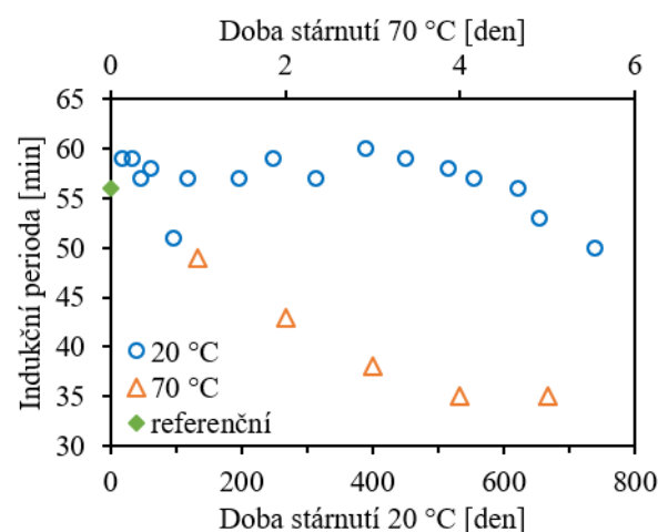
Obr. 10 Závislost indukční periody vzorku č. 4 z PP na době dlouhodobého skladování při 20 °C a akcelerovaného stárnutí při 70 °C
