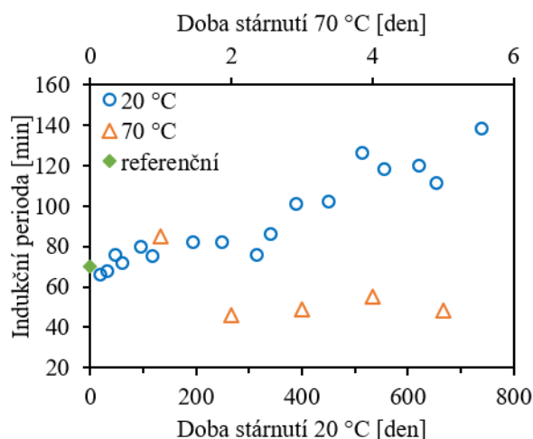
Obr. 11 Závislost indukční periody vzorku č. 5 z polyolefinů na době dlouhodobého skladování při 20 °C a akcelerovaného stárnutí při 70 °C
