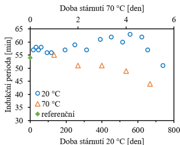
Obr. 13 Závislost indukční periody vzorku č. 7 z polyolefinů na době dlouhodobého skladování při 20 °C a akcelerovaného stárnutí při 70 °C
