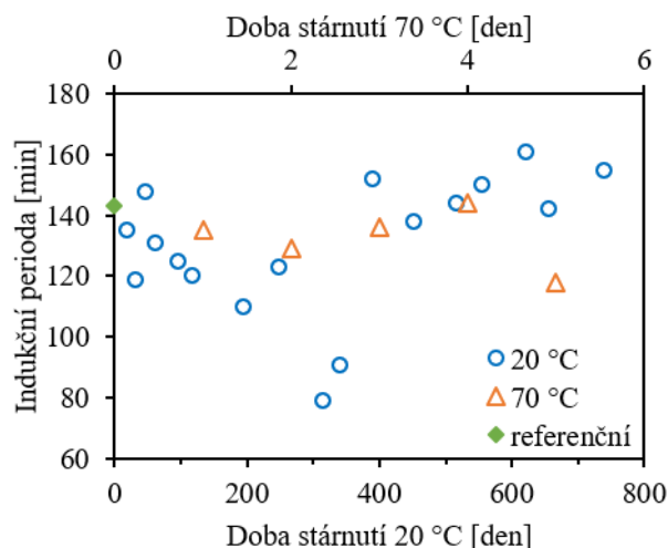
Obr. 9 Závislost indukční periody vzorku č. 3 z pneumatik na době dlouhodobého skladování při 20 °C a akcelerovaného stárnutí při 70 °C Fig. 9 The dependence of the induction period of pyrolysis oil No. 3 from polyolefins on the duration of long-term storage at 20 °C and accelerated aging at 70 °C
