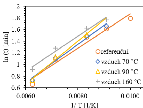
Obr. 4 Teplotní závislost indukční periody podle Arrheniovy rovnice vzorku č. 1 z polyolefinů stárnutého za různých teplot v přítomnosti vzduchu Fig. 4 Temperature dependence of the induction period, as described by the Arrhenius equation, for pyrolysis oil No. 1 derived from polyolefins aged at various temperatures in the presence of air
