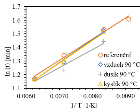
Obr. 6 Teplotní závislost indukční periody podle Arrheniovy rovnice vzorku č. 2 z pneumatik stárnutého při 90 °C v atmosféře vzduchu, dusíku a kyslíku Fig. 6 Temperature dependence of the induction period, as determined by the Arrhenius equation, for pyrolysis oil No. 2 derived from tires aged at 90 °C in an atmosphere of air, nitrogen, and oxygen
