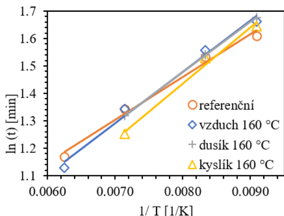
Obr. 7 Teplotní závislost indukční periody podle Arrheniovy rovnice vzorku č. 2 z pneumatik stárnutého při 160 °C v atmosféře vzduchu, dusíku a kyslíku Fig. 7 Temperature dependence of the induction period, as determined by the Arrhenius equation, for pyrolysis oil No. 2 derived from tires aged at 160 °C in an atmosphere of air, nitrogen, and oxygen
