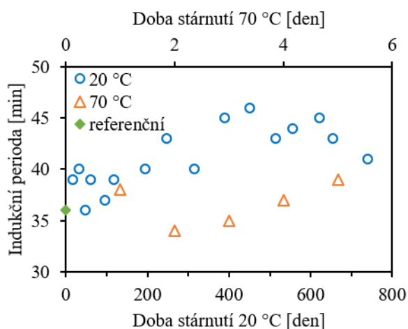
Obr. 12 Závislost indukční periody vzorku č. 6 z polyolefinů na době dlouhodobého skladování při 20 °C a akcelerovaného stárnutí při 70 °C
