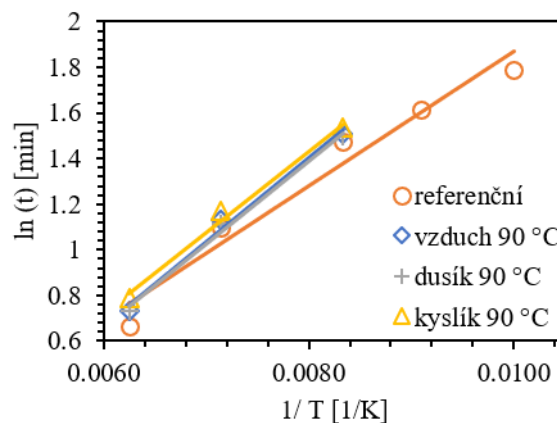
Obr. 2 Teplotní závislost indukční periody podle Arrheniovy rovnice vzorku č. 1 z polyolefinů stárnutého při teplotě 90 °C v atmosféře vzduchu, dusíku a kyslíku Fig. 2 Temperature dependence of the induction period, as determined by the Arrhenius equation, for pyrolysis oil No. 1 derived from polyolefins aged at 90 °C in an atmosphere of air, nitrogen, and oxygen
