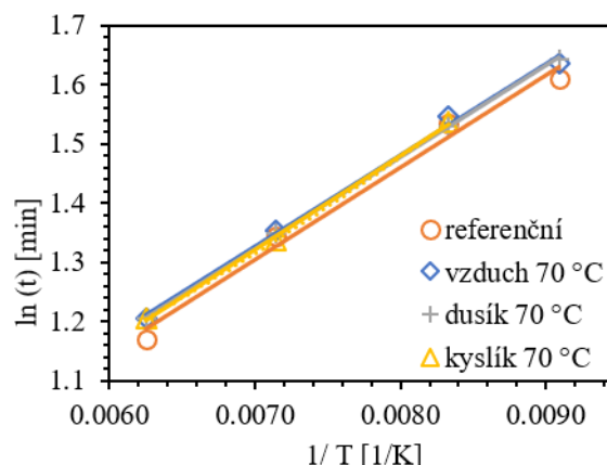
Obr. 5 Teplotní závislost indukční periody podle Arrheniovy rovnice vzorku č. 2 z pneumatik stárnutého při 70 °C v atmosféře vzduchu, dusíku a kyslíku Fig. 5 Temperature dependence of the induction period, as determined by the Arrhenius equation, for pyrolysis oil No. 2 derived from tires aged at 70 °C in an atmosphere of air, nitrogen, and oxygen
