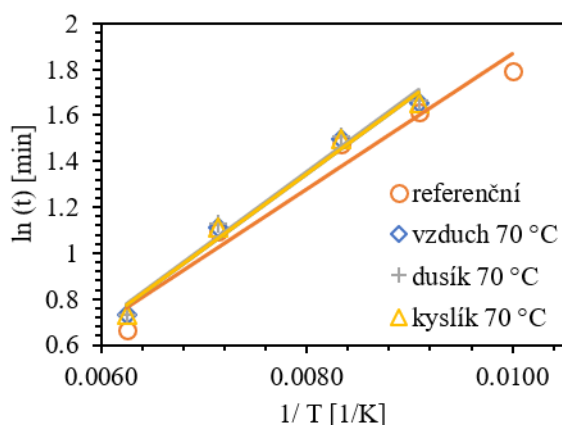
Obr. 1 Teplotní závislost indukční periody podle Arrheniovy rovnice vzorku č. 1 z polyolefinů stárnutého při teplotě 70 °C v atmosféře vzduchu, dusíku a kyslíku Fig. 1 Temperature dependence of the induction period, as determined by the Arrhenius equation, for pyrolysis oil No. 1 derived from polyolefins aged at 70 °C in an atmosphere of air, nitrogen, and oxygen
