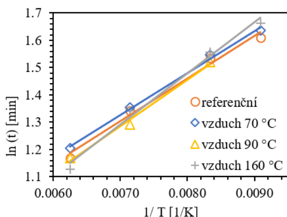
Obr. 8 Teplotní závislost indukční periody podle Arrheniovy rovnice vzorku č. 2 z pneumatik stárnutého za různých teplot v přítomnosti vzduchu Fig. 8 Temperature dependence of the induction period, as described by the Arrhenius equation, for pyrolysis oil No. 2 derived from tires aged at various temperatures in the presence of air
