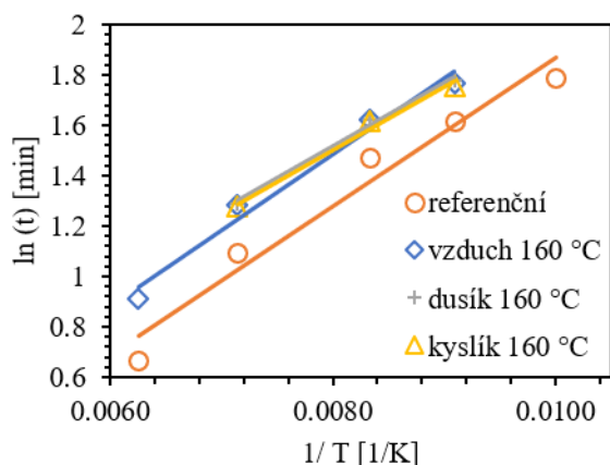
Obr. 3 Teplotní závislost indukční periody podle Arrheniovy rovnice vzorku č. 1 z polyolefinů stárnutého při teplotě 160 °C v atmosféře vzduchu, dusíku a kyslíku Fig. 3 Temperature dependence of the induction period, as determined by the Arrhenius equation, for pyrolysis oil No. 1 derived from polyolefins aged at 160 °C in an atmosphere of air, nitrogen, and oxygen
